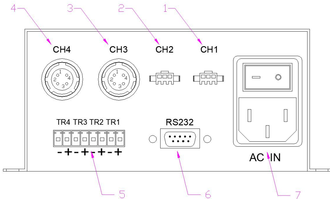
图 2 后面板各部件功能示意图
