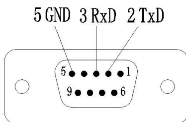
图 5 RS232 插头示意图
