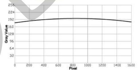
光谱图
