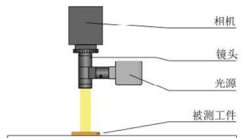
点光源打光示意图
