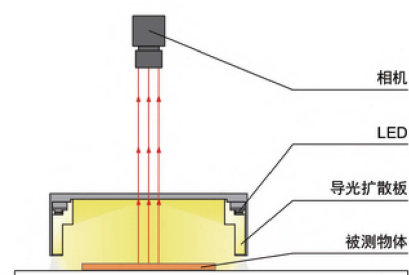
散射型方形光源打光示意图
