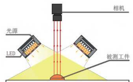
条形光源打光示意图
